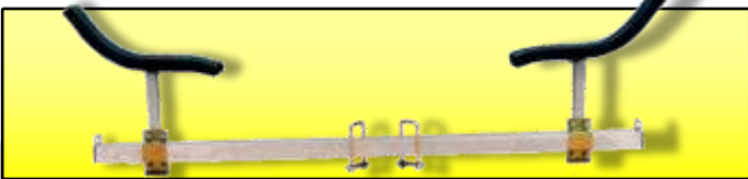
Ensemble composé de :- une traverse Réf.:11041 - 2 patins latéraux Réf.:11010 - brides et omégas
